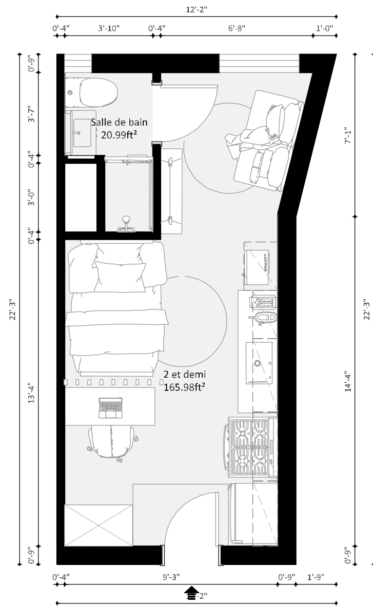
Plan Complet 1:50
