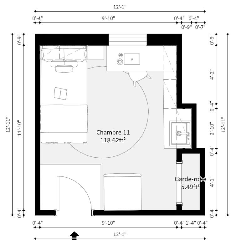
Plan Complet 1:50
